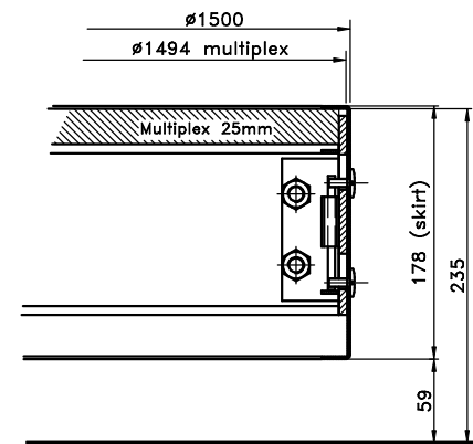
detail A M 1:1
