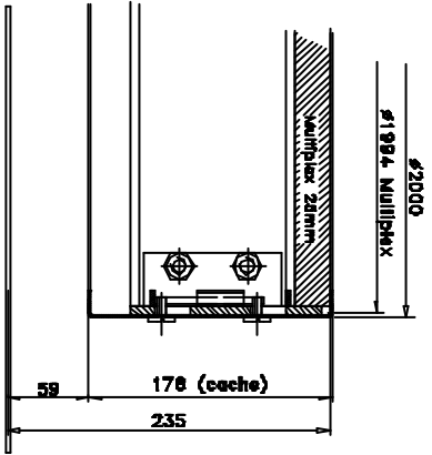
détail A M 1:1
